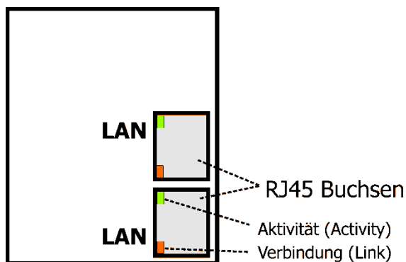
CM-Modbus/TCP-2P
